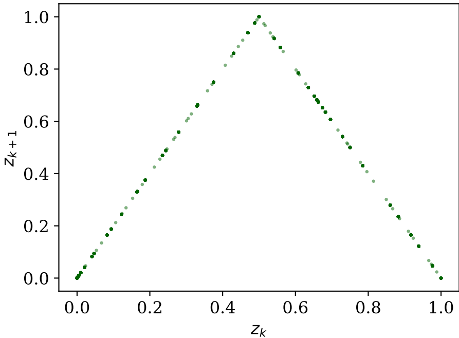
Диаграмма возвратов ( z_{k+1} от z_k )
